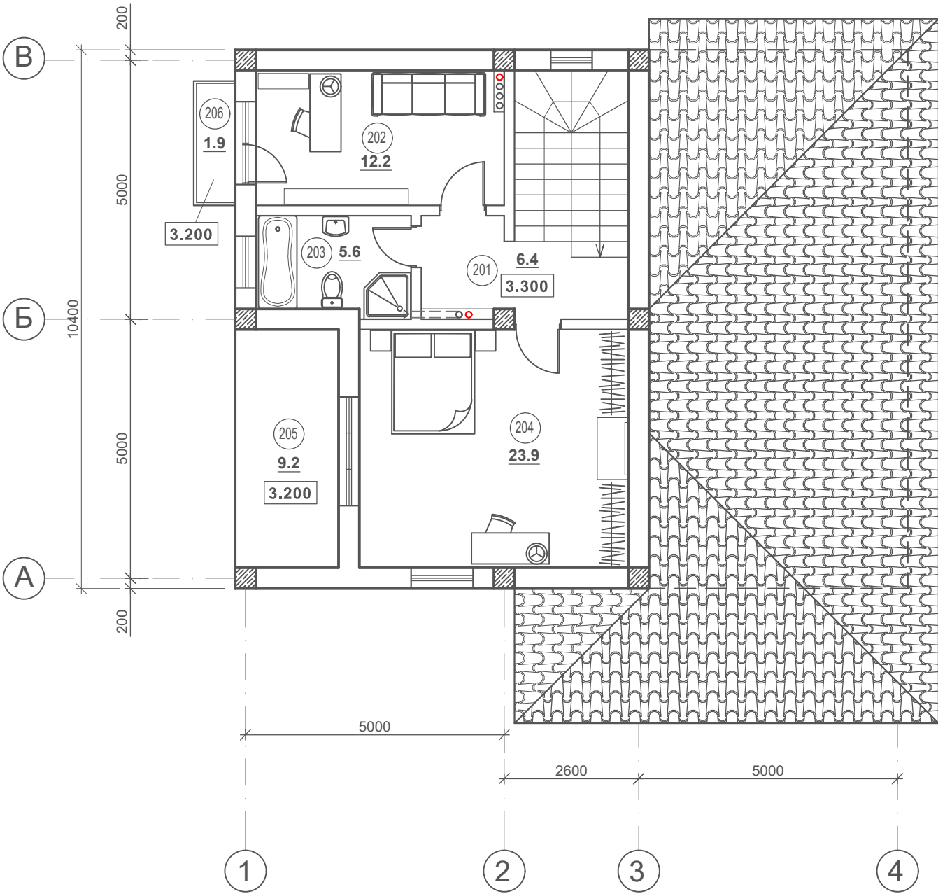
План расстановки мебели и оборудования второго этажа
